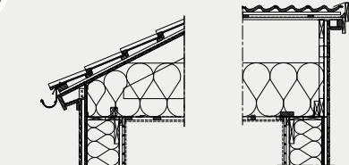
Kort takfot
