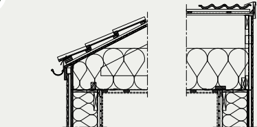
Ingen takfot
