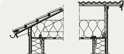
Mellanlång takfot
